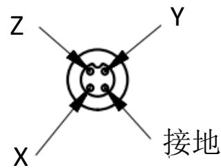
四芯连接器
